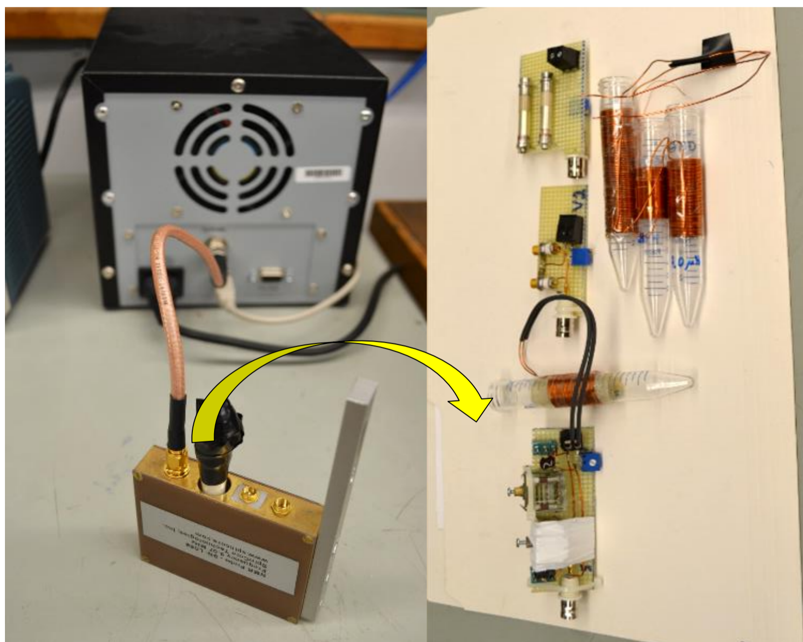
Figure 1 : Système NQR bâti sur mesure pour la détection de composés renfermant de l'azote (p. ex., drogues, explosifs) La flèche indique une sonde d'échantillonnage
