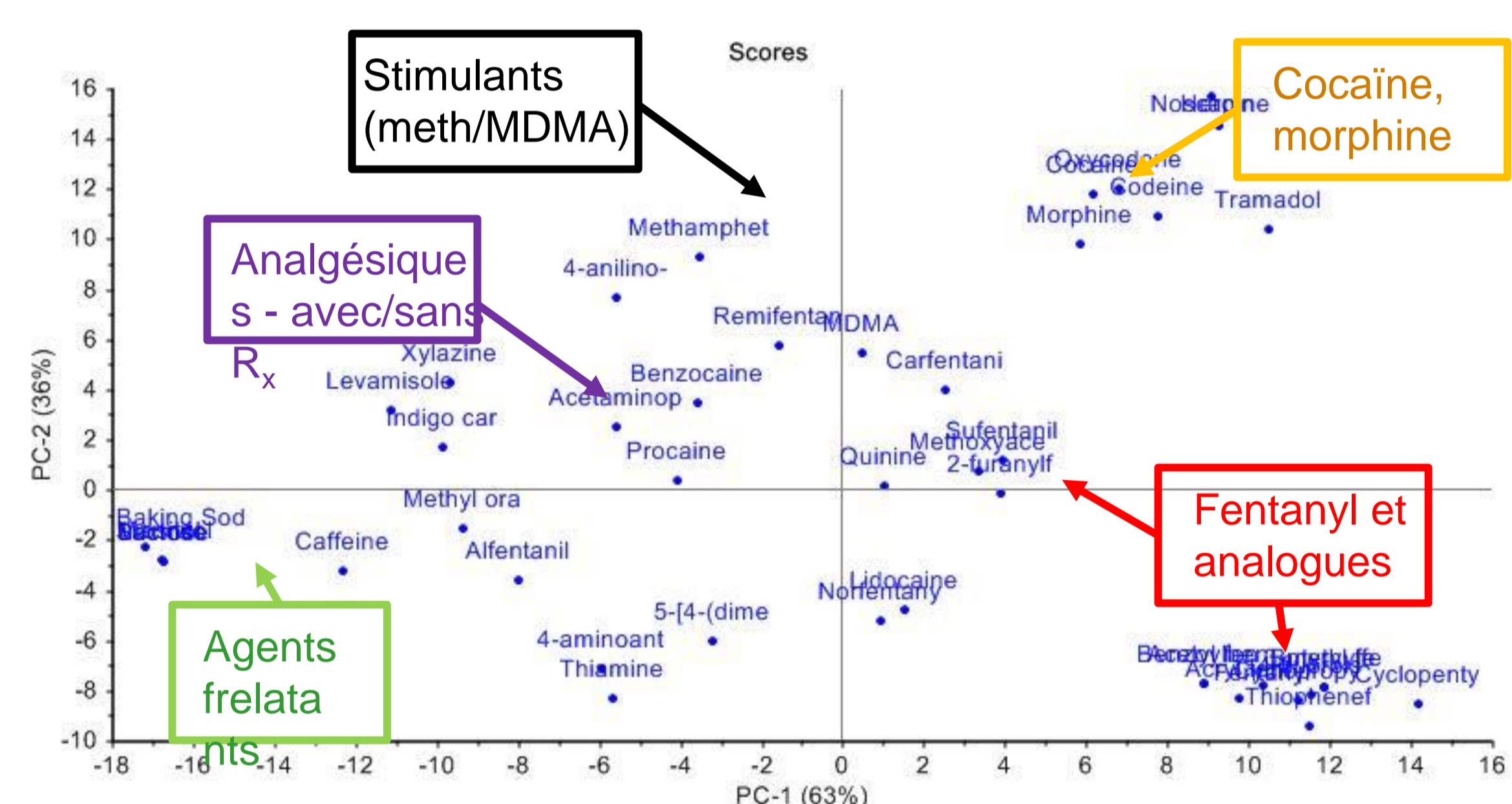
Figure 3 : Graphique de l'analyse de composante principale de drogues et de médicaments d'ordonnance et de la majorité des agents frelatants selon un modèle de rapport atomique des molécules dans la forme pure.
