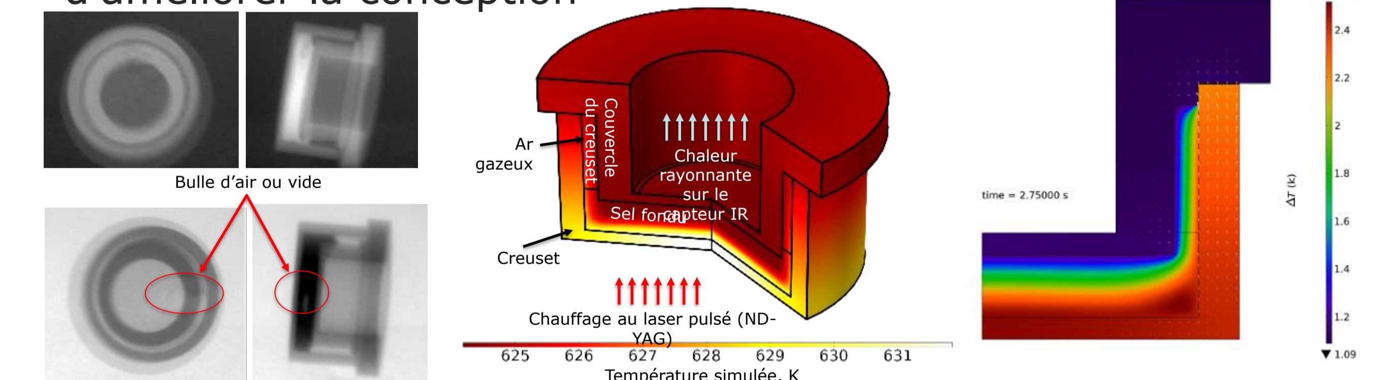
Figure : Radiographie du sel de nitrate dans le support d'échantillon de graphite et résultats de FEM
