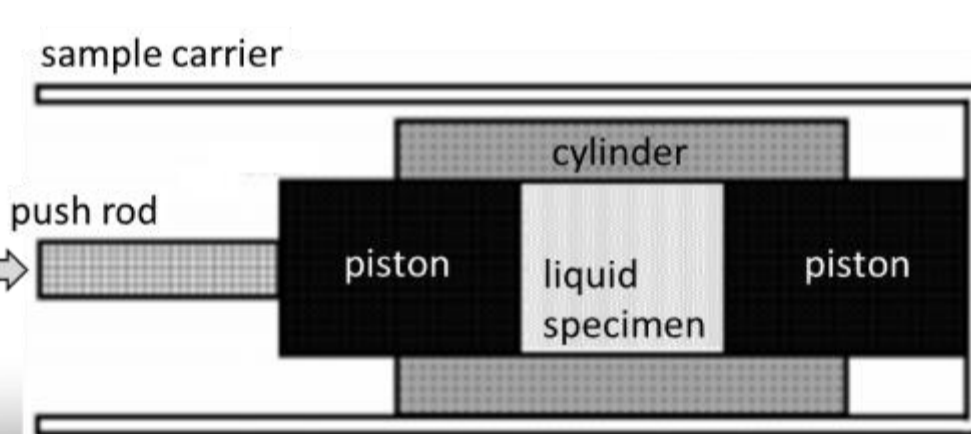
Figure : Appareil utilisé pour évaluer les mesures dilatométriques de la densité du sel de nitrate (Netzsch 402C/7)
